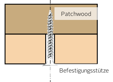
Schraubmontage
